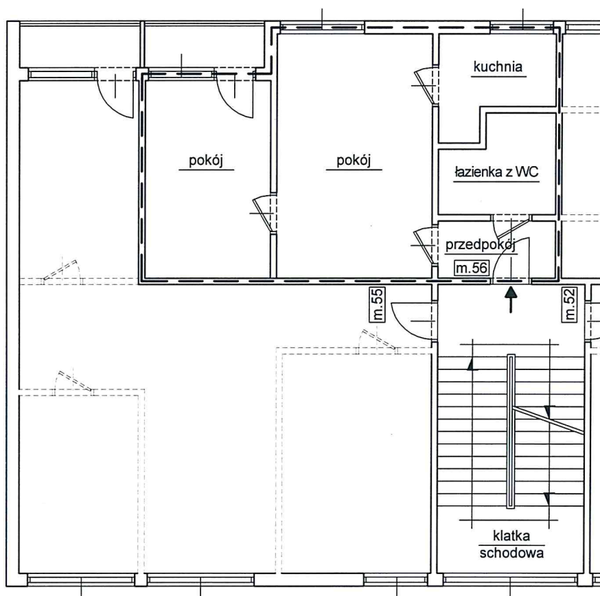
Rzut III-go piętra - fragment
